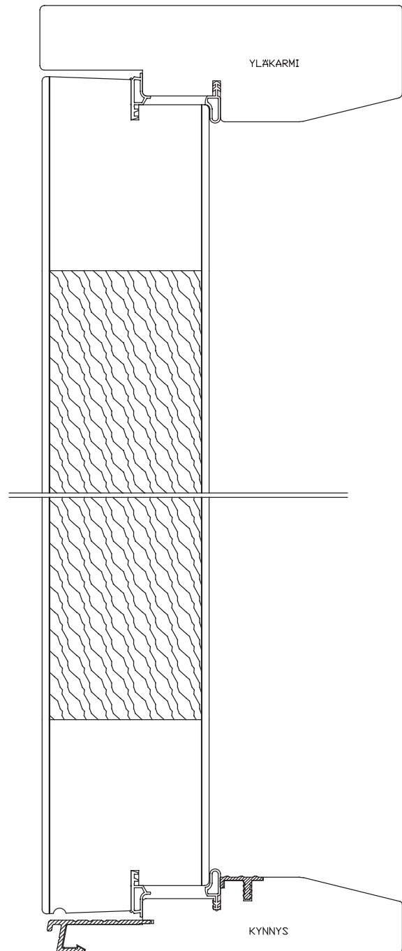
Pystyleikkaus, umpiovi
