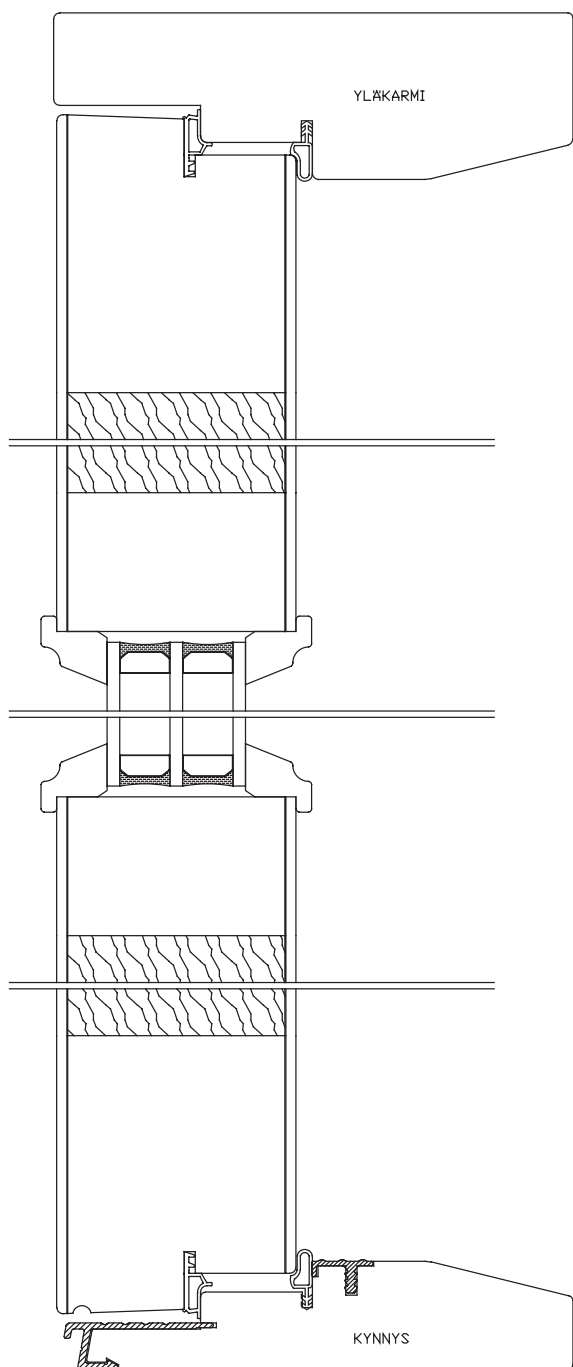
Pystyleikkaus, lasiaukollinen ulko-ovi
