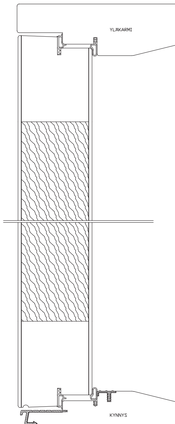
Pystyleikkaus, umpiovi
