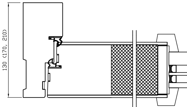
Vaakaleikkaus lasiosa
