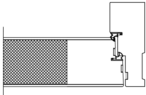
Vaakaleikkaus eristeosa
