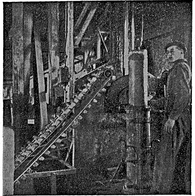
TANSKALAINEN APOLLO-PUTKENSULLOJA, johon koneellisen sullonnan lisäksi on yhdistetty tärypöytä, valmistaa vesitiiviitä, kestäviä putkia.
