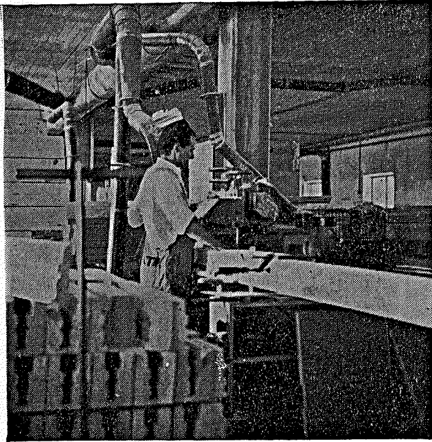
RUOTSALAINEN JONSEREDS-TAPPIKONE. Karmien tapitus käynnissä.
